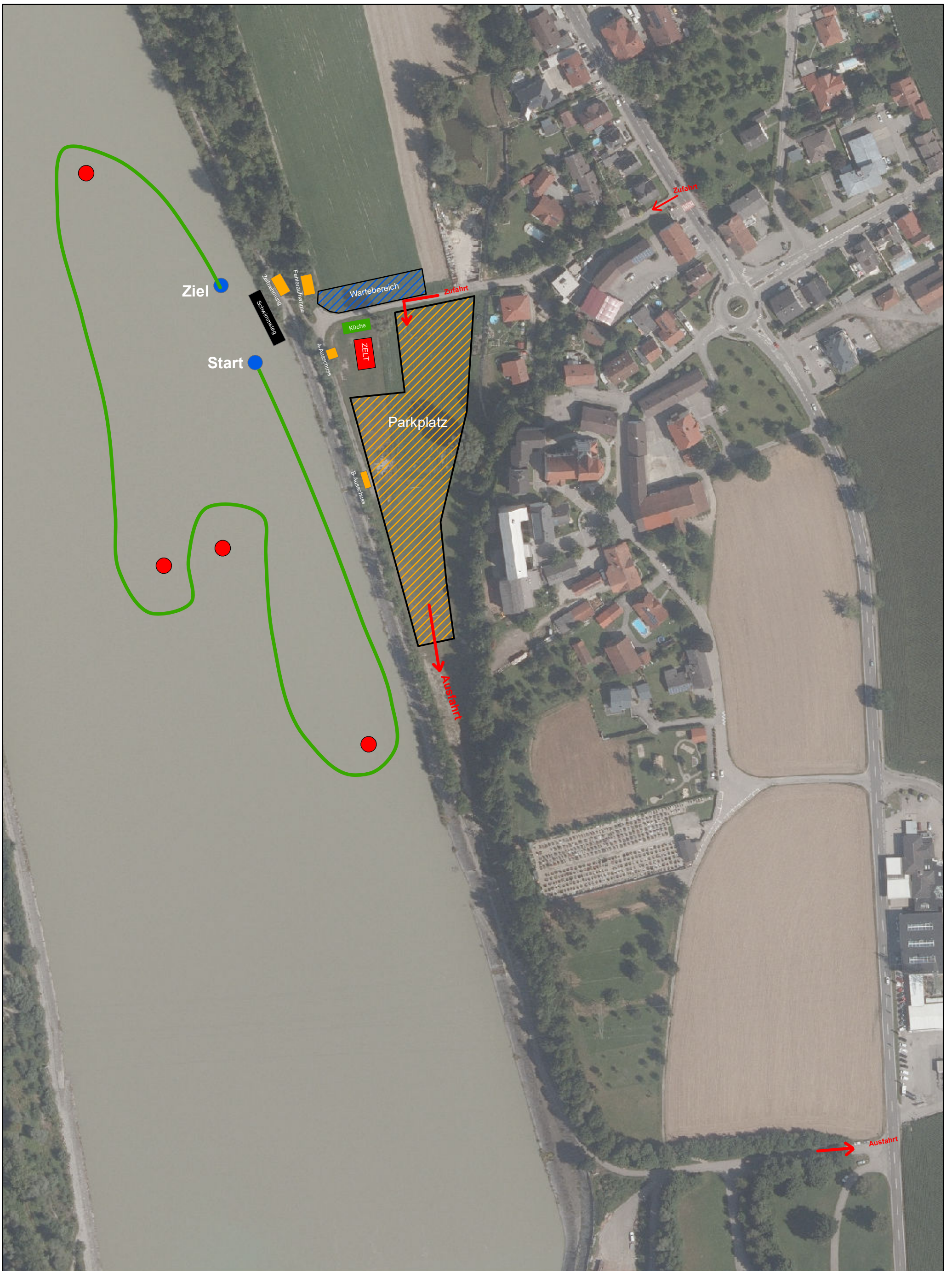
Landeswasserwehrbewerb St. Florian am Inn Übersichtsplan
